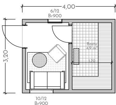
Bastu Modul
